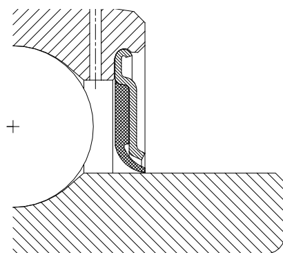
Рис. 8: уплотнение корпусных подшипников NKE типа P.
