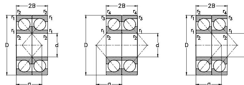
X-Anordnung Face to face arrangement
