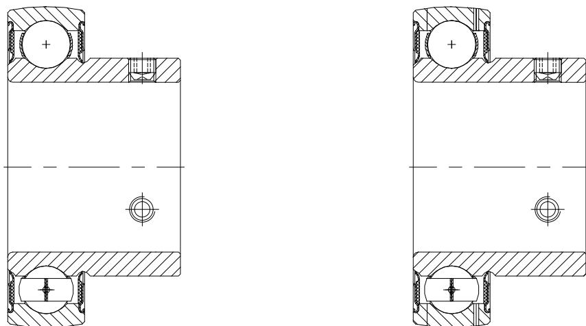
Рис. 4: корпусные подшипники NKE конструкций AY и GAY
