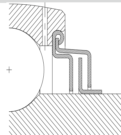
Рис. 11: уплотнение типа L для корпусных подшипников NKE
